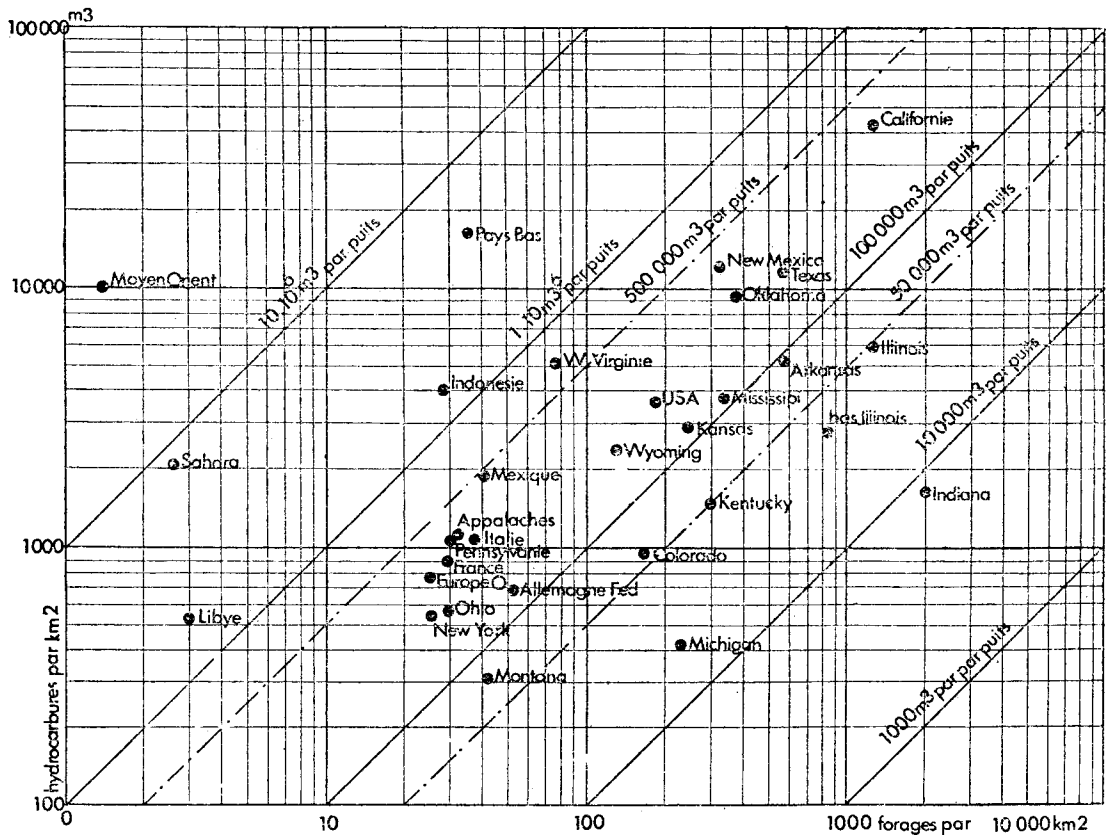
شکل ۱۱ - مقدار ئیدروکربور کشف شده در کیلومتر مربع بر حسب دانستیه حفاری
