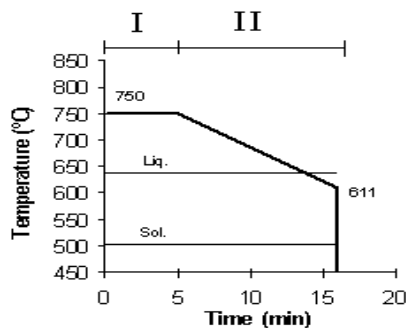
شکل ۱: سیکل مورد استفاده جهت تولید مخلوط پودری Al_2O_3/Gr .
