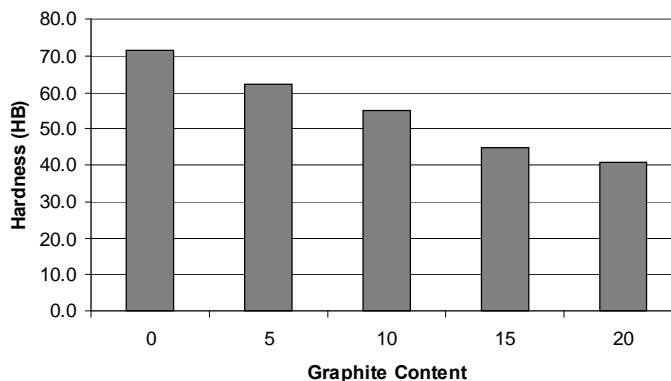
شکل ۳: تغییرات سختی نمونه های کامپوزیتی Al_{20}Gr با تغییر محتوای گرافیت.
